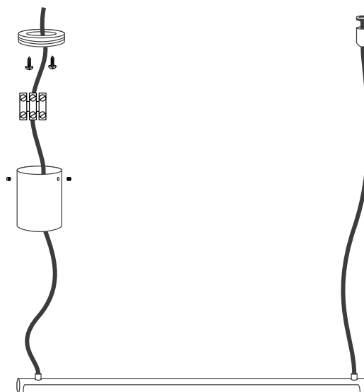
Рис. 2. Установка и подключение светильника
