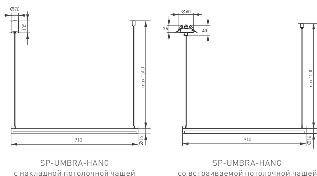
Рис. 1. Чертеж и габаритные размеры
