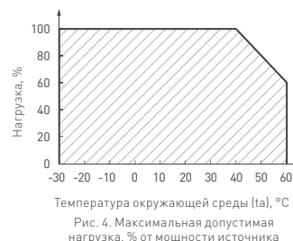
Рис. 4. Максимальная допустимая нагрузка, % от мощности источника
