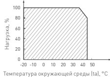
Рис. 2. Максимальная допустимая нагрузка, % от мощности источника
