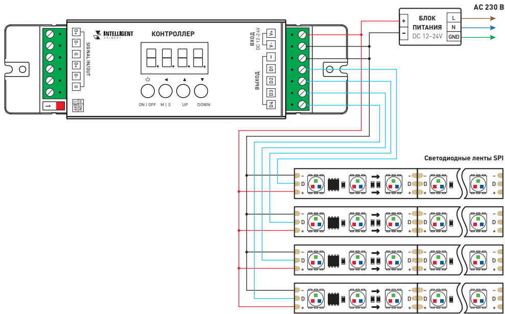
Рис. 2. Схема подключения контроллера
