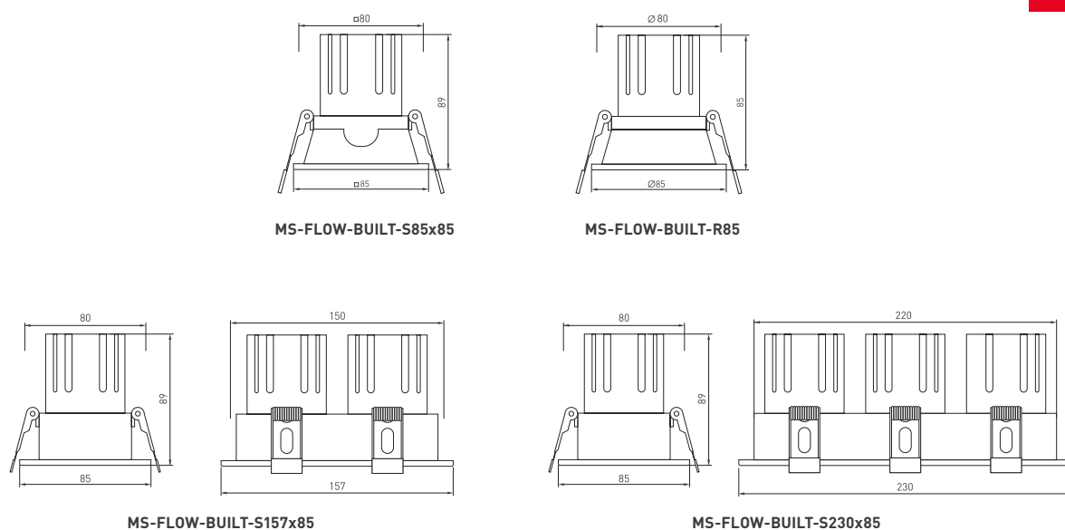
Рис. 1. Чертеж и габаритные размеры
