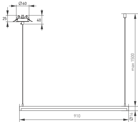
SP-UMBRA-HANG со встраиваемой потолочной чашей
