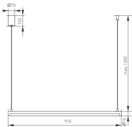
SP-UMBRA-HANG с накладной потолочной чашей
