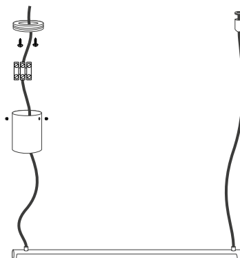
Рис. 2. Установка и подключение светильника
