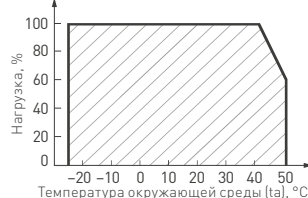
Рис. 5. Максимальная допустимая нагрузка, % от мощности источника
