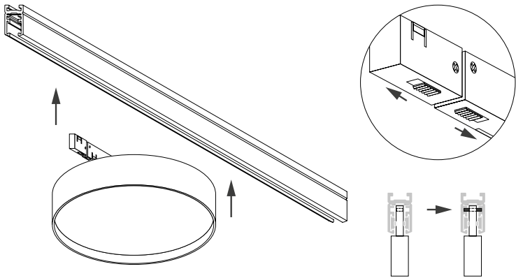
Рис. 2. Установка светильника
