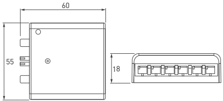
Рис. 1. Габаритный чертеж
