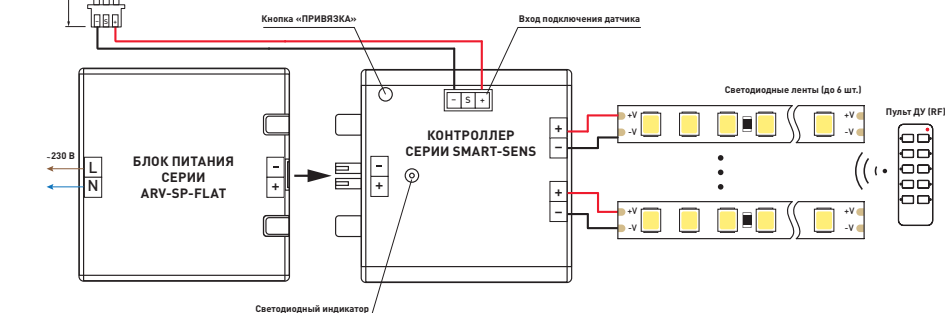
Рис. 3. Схема подключения контроллера к блокам питания серии ARV-SP-FLAT
