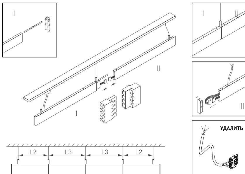
Рис. 3. Соединение светильников в линию
