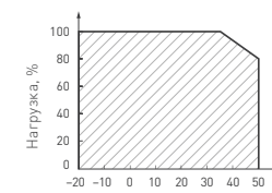
Рис. 2. Максимальная допустимая нагрузка, % от мощности источника
