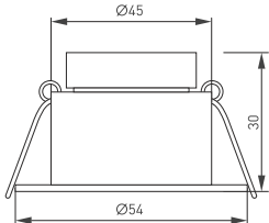
Рис. 1. Чертеж и габаритные размеры
