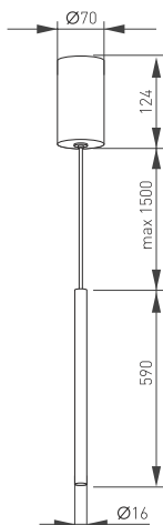
SP-UMBRA-HANG с накладной потолочной чашей
