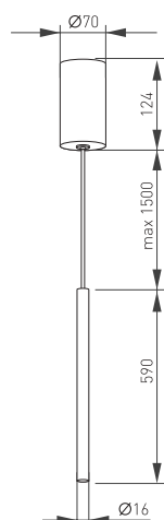
SP-UMBRA-HANG с накладной потолочной чашей
