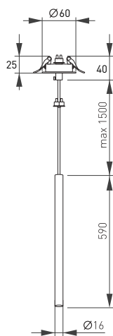
SP-UMBRA-HANG со встраиваемой потолочной чашей
