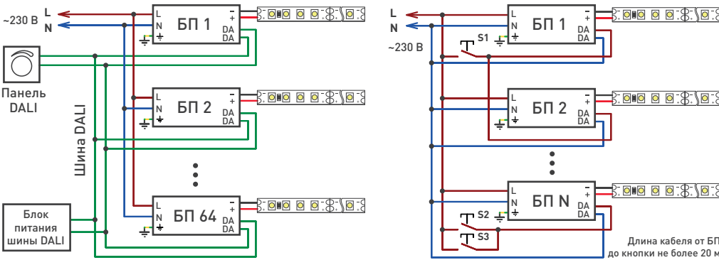
Рис. 2. Структурная схема соединения оборудования при использовании управления DALI
